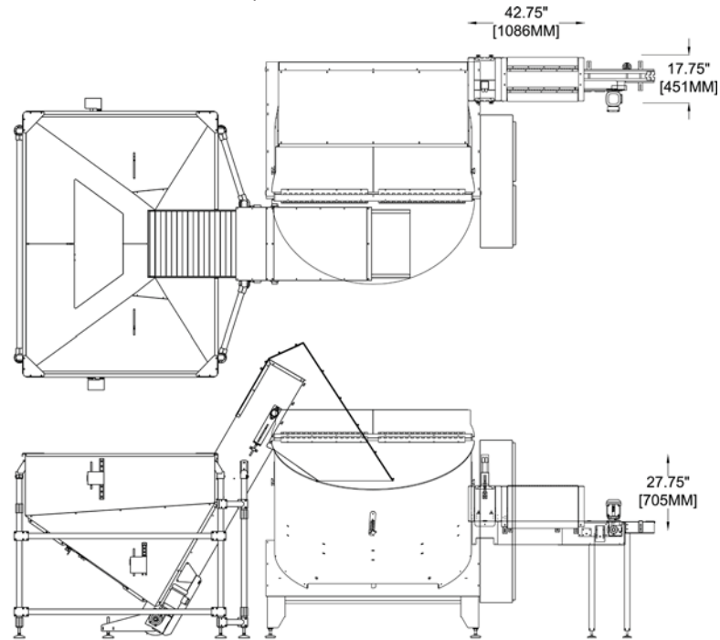
NECO-ORIENTER 180 integrada con posicionadores de Botellas
